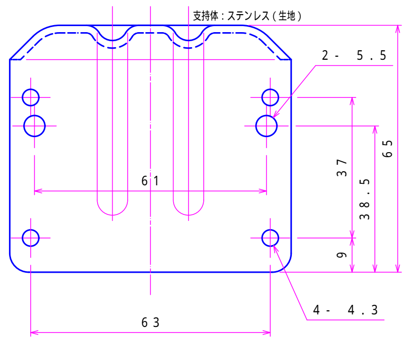
矢視 A
