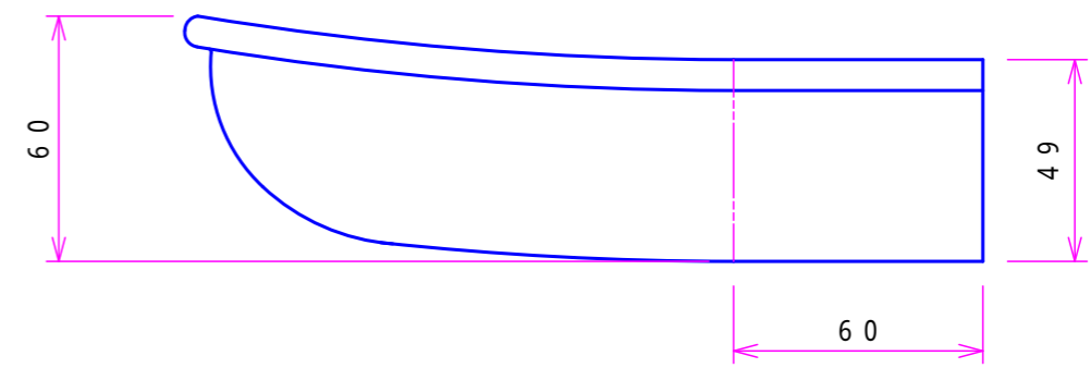
側面図 ( 1 / 2 )
