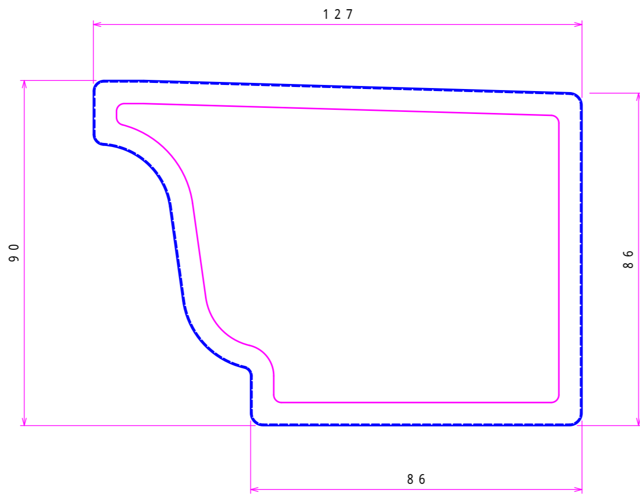
水止め (右)
